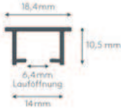
Querschnitt HM110
